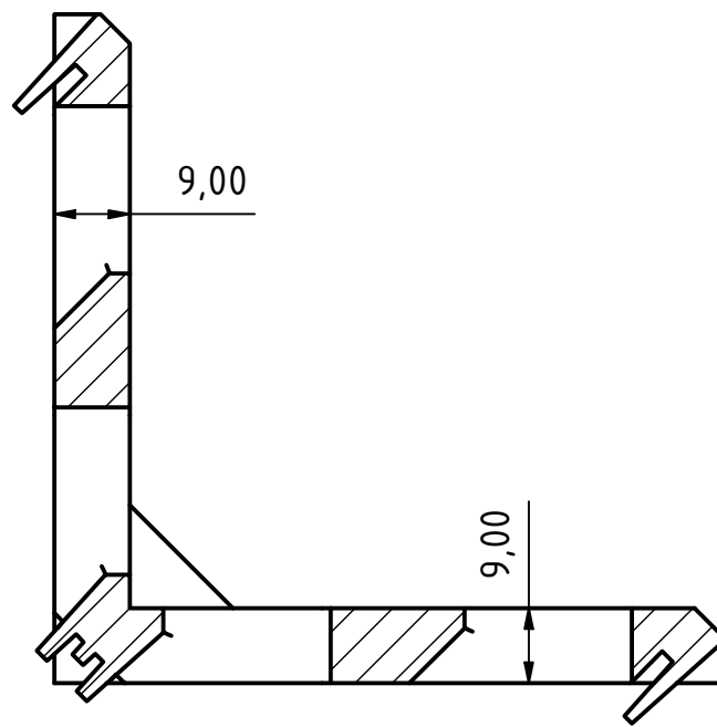
A-A ( 1 : 1 ) / .
