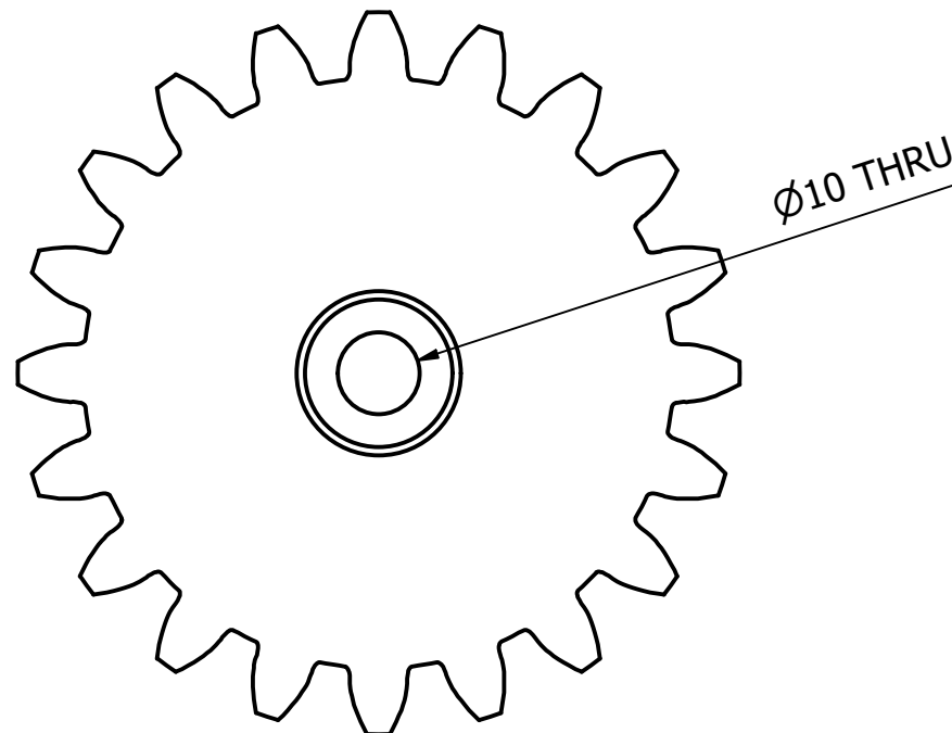
VIEW1 ( 1:1 )
