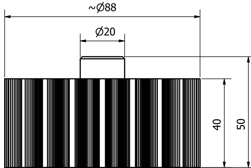
VIEW1 ( 1:1 )
