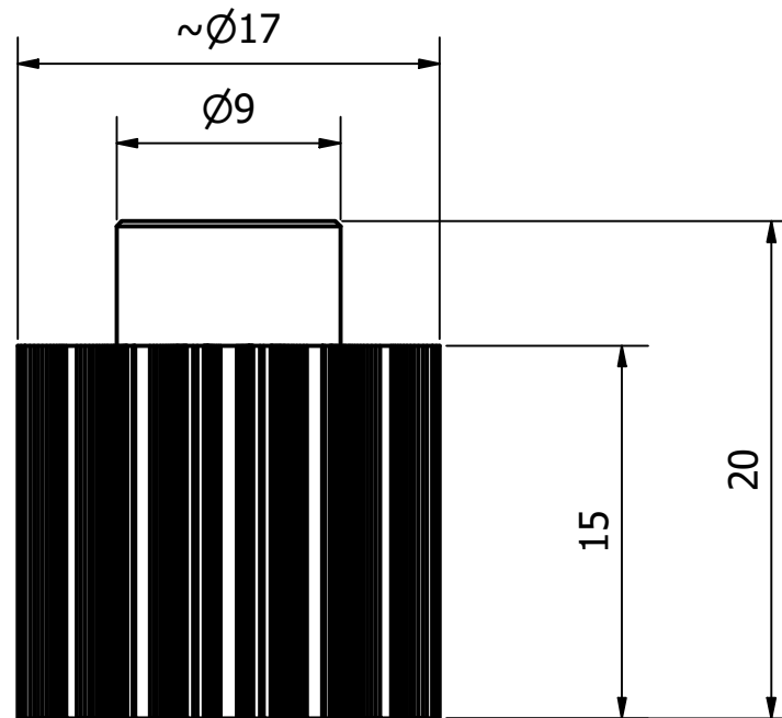
VIEW1 ( 3 : 1 )
