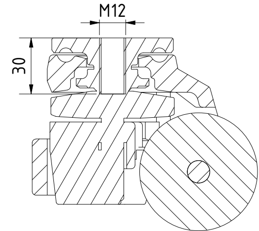
A-A ( 1 : 2 ) / .
