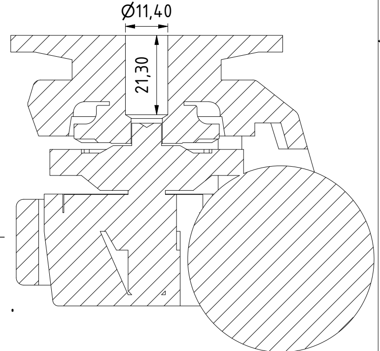
A-A ( 1 : 1 ) / .
